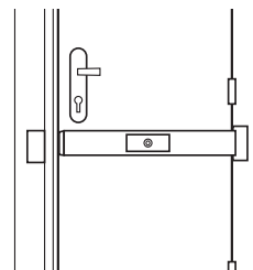
Querriegelschloss
