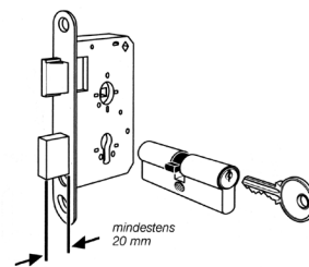
Türschloss
